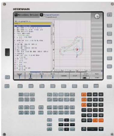
TNC 620 mit Bedientasten
